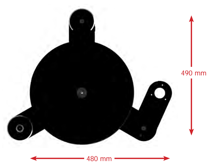
Abb. 3: Aufstellfläche Innovation Basic
