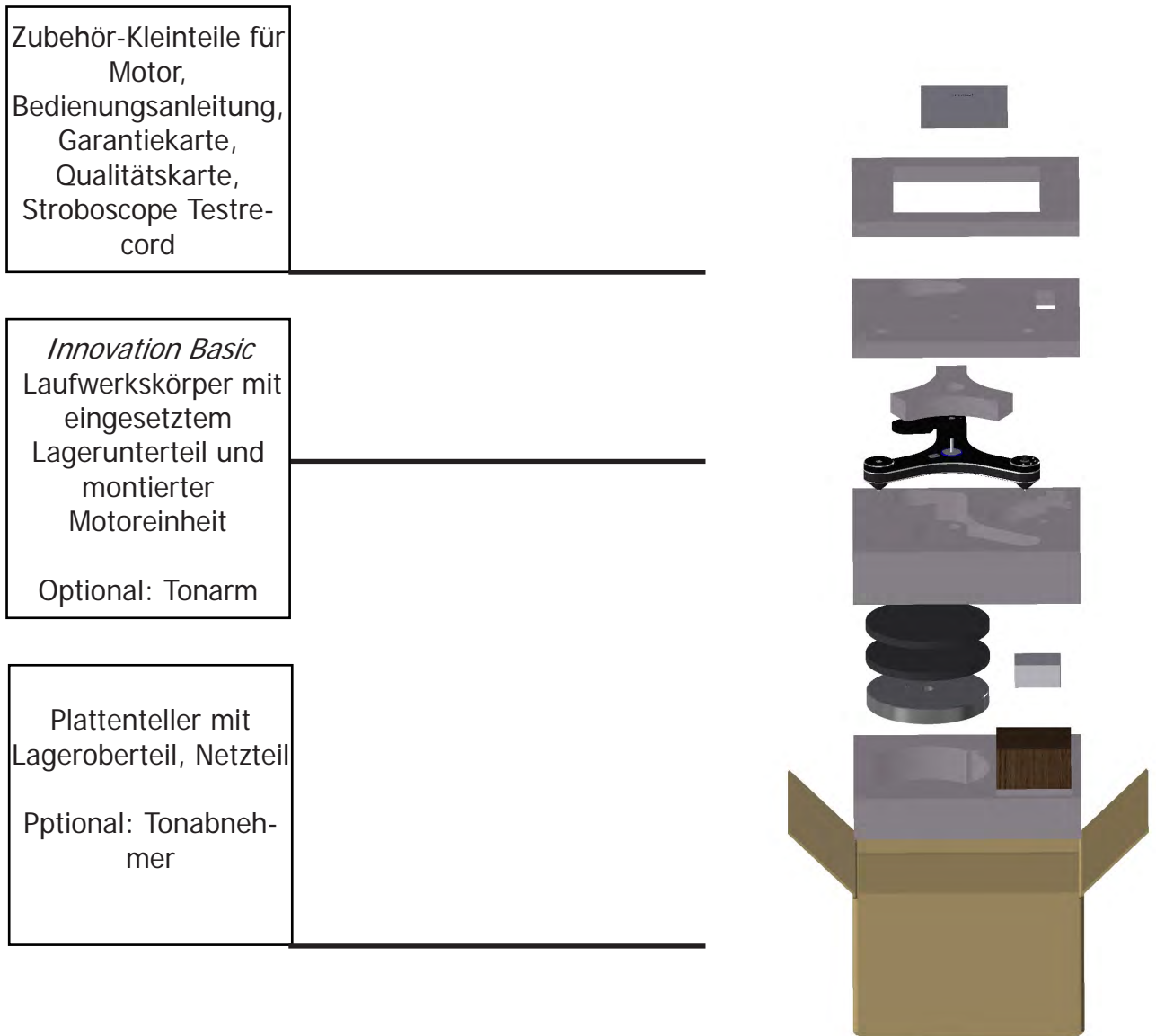
Abb. 1: Verpackungsübersicht
